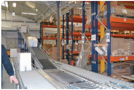
Système de circulation et gare n° 20 .
