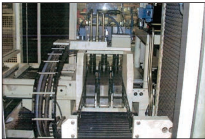
Poinçonnage en ligne (Dallan, Italie).
